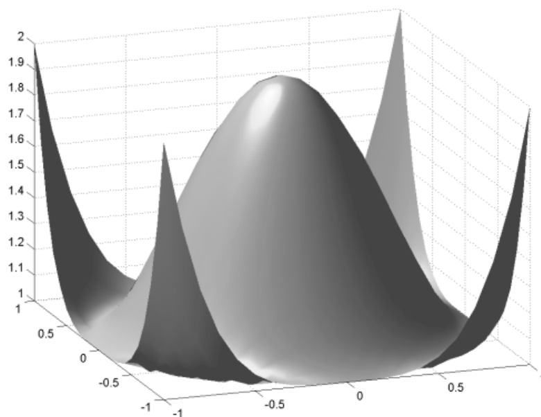
Rysunek 1: Wykres f(x, y) = x^4 + y^4 + 2(x - 1)(x + 1)(y - 1)(y + 1) dla (x, y) \in [-1, 1] \times [-1, 1] .
