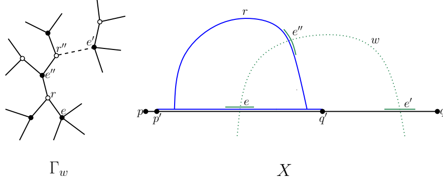
FIGURE 7. Lemma 5.1.
