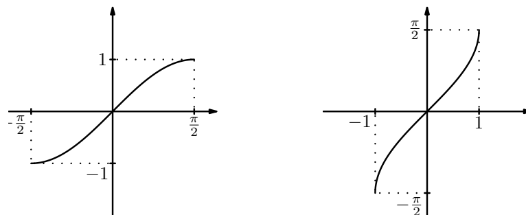
Rysunek 7.2: Funkcja \sin(x) i \arcsin(x) .
