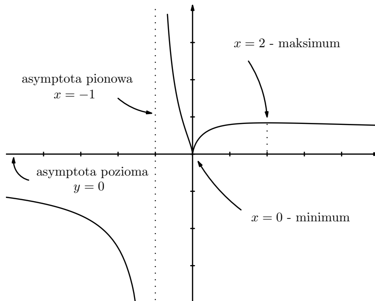
Rysunek 8.7: Wykres funkcji z przykładu (c).
