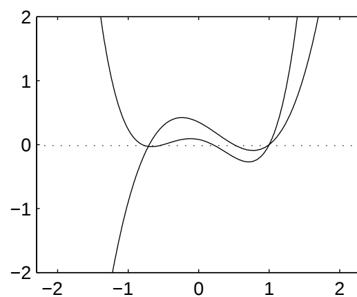
Rysunek 3.1: Przykładowe wielomiany stopnia 3 i 4.
