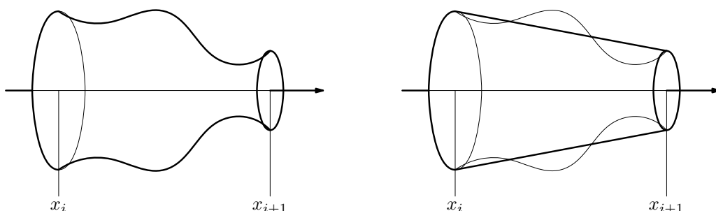
Rysunek 11.7: Stożek przybliżający bryłę obrotową.
