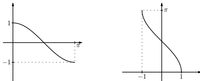
Rysunek 7.3: Funkcja \cos(x) i \arccos(x) .
