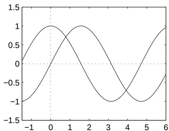
Rysunek 3.6: Funkcje \sin(x) i \cos(x) .
