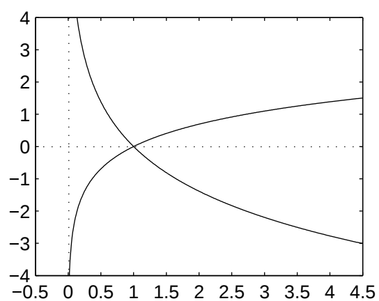
Rysunek 3.5: Logarytmy, o podstawach mniejszej i większej od 1.
