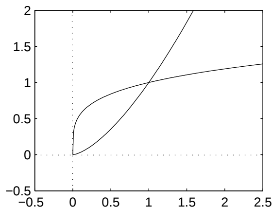
Rysunek 3.3: Dwie funkcje potęgowe, z wykładnikami 0,25 i 1,5.
