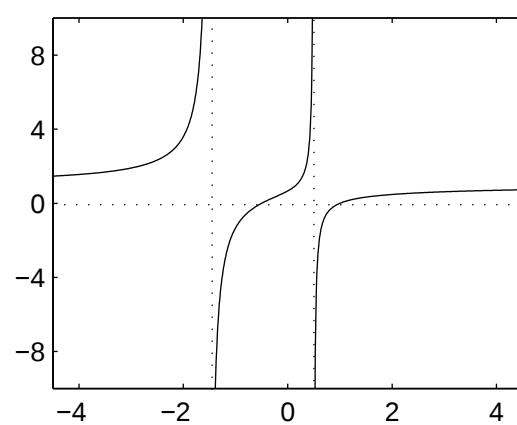
Rysunek 3.2: Przykład funkcji wymiernej.
