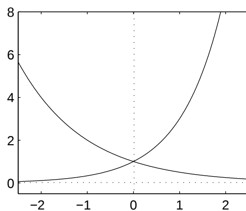
Rysunek 3.4: Funkcje wykładnicze o podstawach mniejszej i większej od 1
