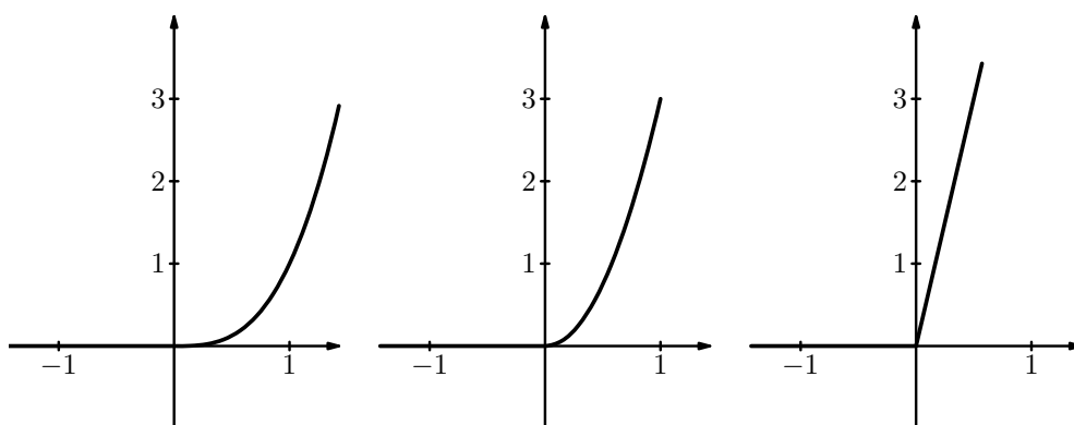
Figure 8.4: Funkcje f , f' i f'' z przykładu (b).
