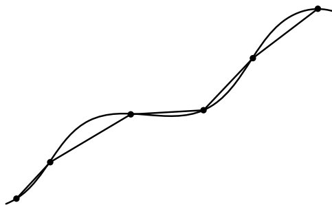
Figure 11.1: Przybliżenie krzywej łamaną.
