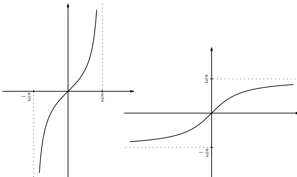
Figure 7.4: Gałąź funkcji \tan(x) i funkcja \arctan(x) .
