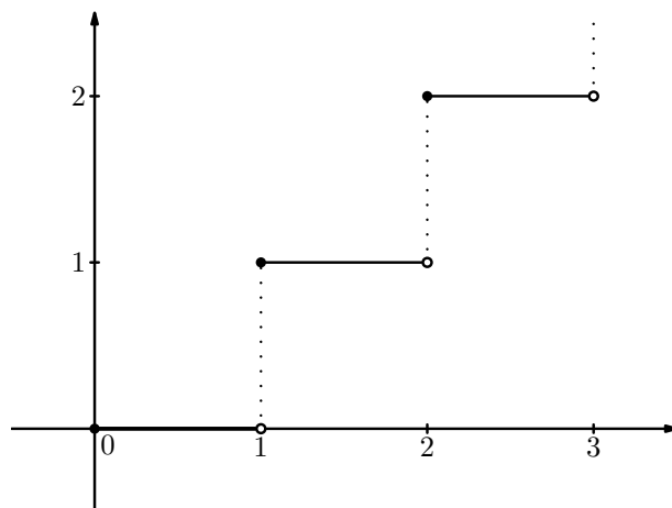
Figure 6.4: Granice jednostronne funkcji [x] .
