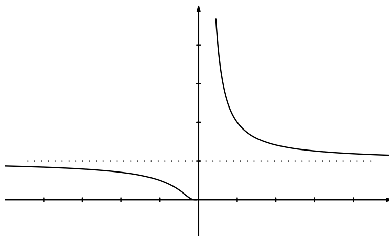
Figure 6.5: Granice w zerze funkcji 2^{\frac{1}{x}} .
