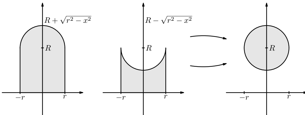
Figure 11.6: Obszar (11.2) jako różnica dwóch obszarów.
