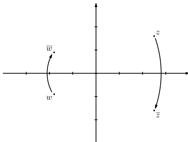
Figure 2.4: Sprzężenie liczby zespolonej
