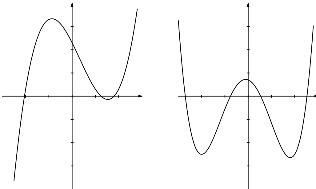
Figure 3.1: Wielomiany stopnia 3 i 4.
