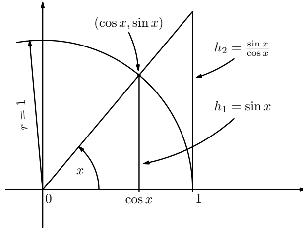
Figure 6.3: Dalsze oszacowanie funkcji \sin(x) .
