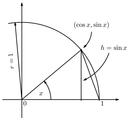
Figure 6.1: Oszacowanie \sin x .
