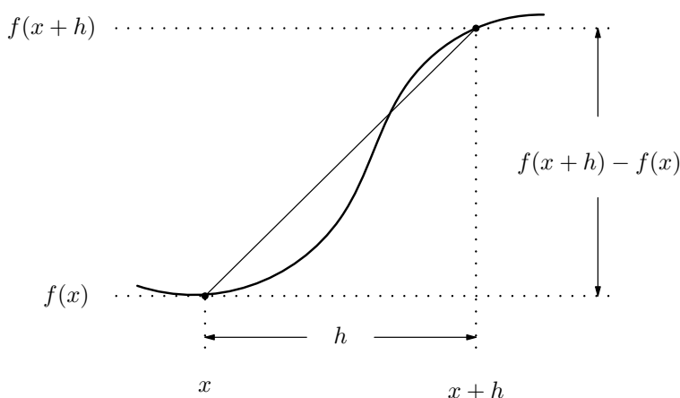
Figure 8.1: Iloraz różnicowy i sieczna wykresu.
