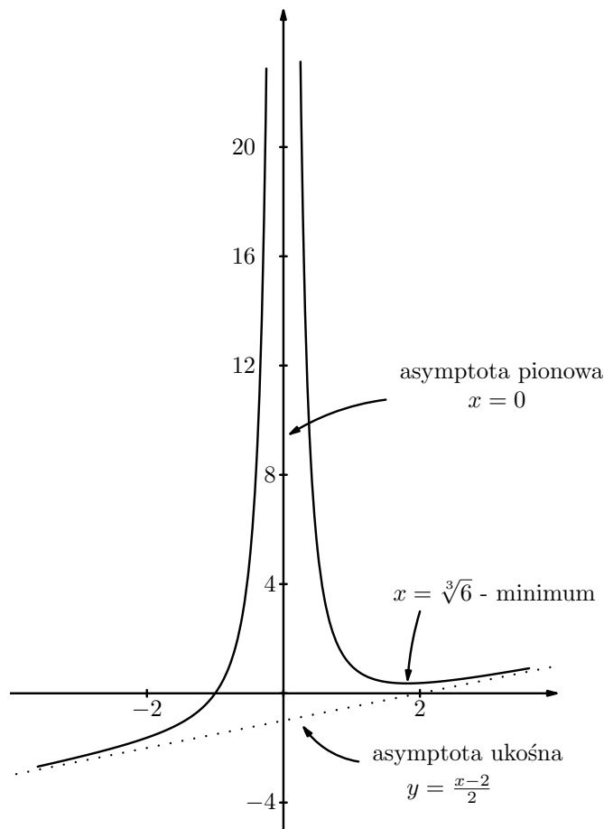
Figure 8.6: Asymptoty funkcji z przykładu (b).
