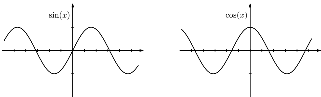
Figure 3.6: Funkcje \sin(x) i \cos(x) .
