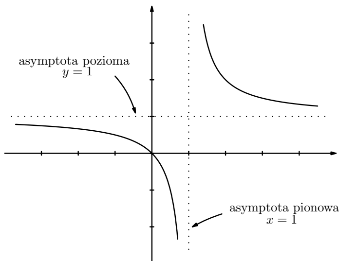
Figure 8.5: Asymptoty funkcji f(x) = \frac{x}{x-1} .
