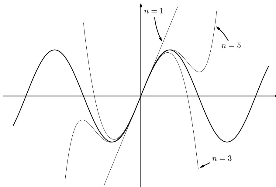
Figure 8.8: Wielomiany Taylora stopnia n funkcji \sin(x) .
