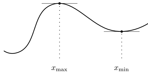
Figure 8.3: Lokalne maksimum i minimum.
