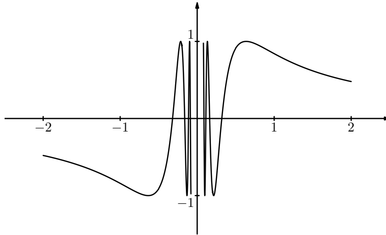
Figure 6.2: Funkcja \sin \frac{1}{x} w otoczeniu 0.
