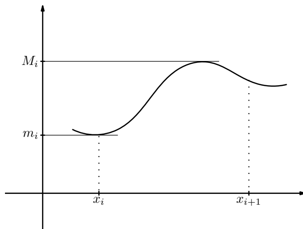
Figure 10.3: m_i oraz M_i .
