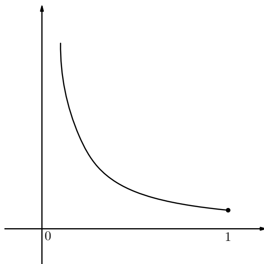
Figure 10.4: Funkcja ciągła, ale nie jednostajnie ciągła.
