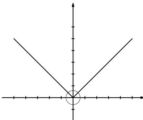
Figure 8.2: Wykres f(x) = |x| i nieróżniczkowalny „dzióbek”.
