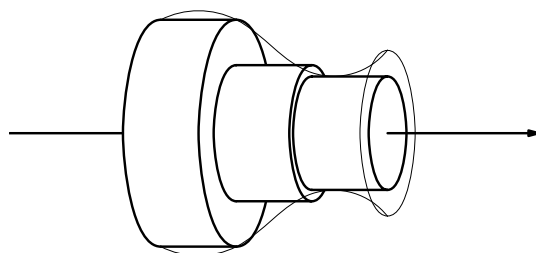
Figure 11.4: Przybliżanie objętości walcami.
