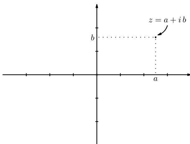
Figure 2.3: Płaszczyzna liczb zespolonych
