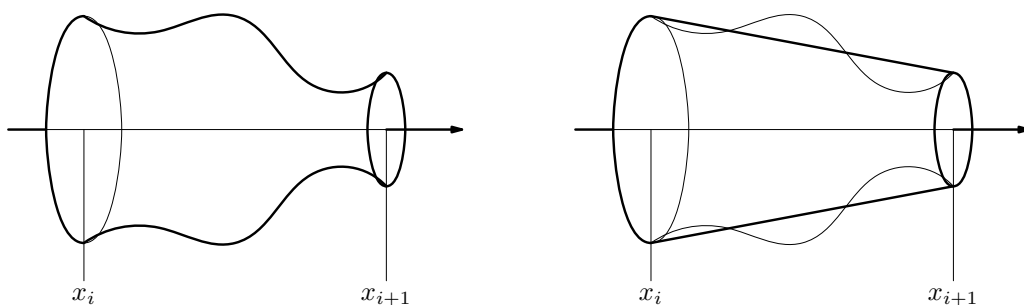
Figure 11.7: Stożek przybliżający bryłę obrotową.
