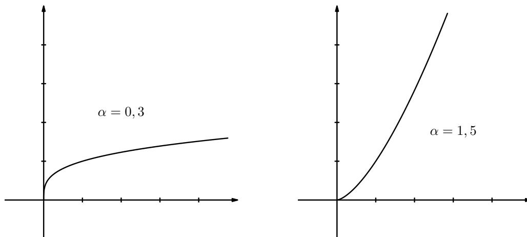
Figure 3.3: Funkcja potęgowa f(x) = x^\alpha .
