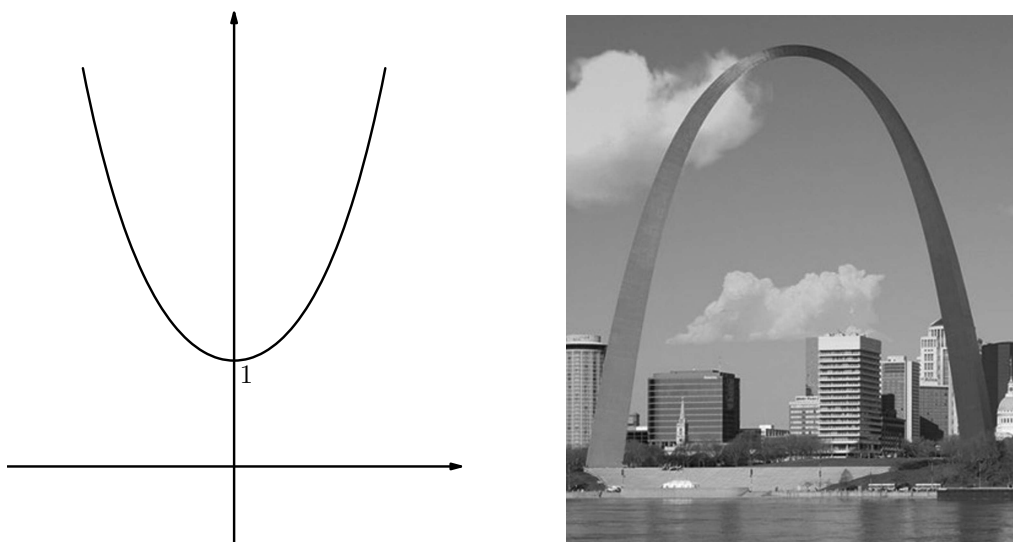
Figure 11.2: Linia łańcuchowa i łuk w St. Louis.
