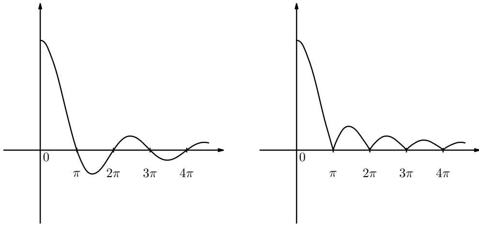
Figure 12.1: Funkcje \frac{\sin x}{x} i \frac{|\sin x|}{x} .
