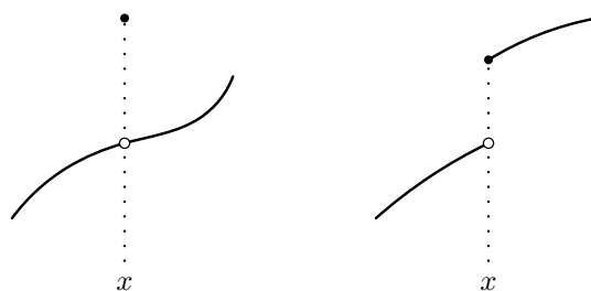
Figure 7.1: Nieciągłość usuwalna i nieciągłość skokowa.
