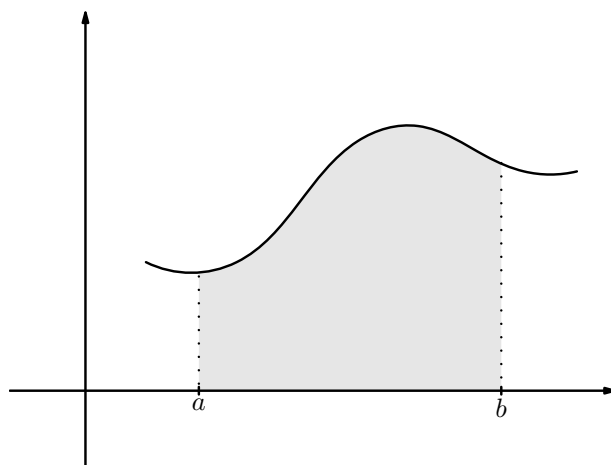
Figure 10.1: Obszar pod wykresem funkcji.
