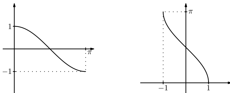
Figure 7.3: Funkcja \cos(x) i \arccos(x) .
