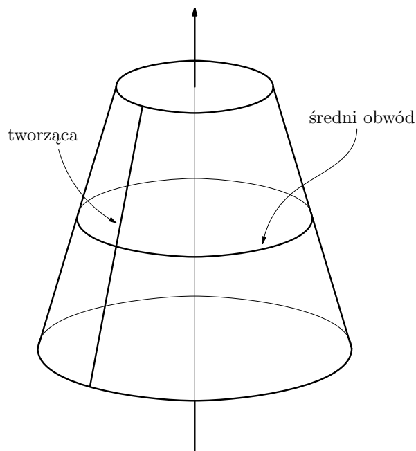
Figure 11.8: Tworząca i średni obwód stożka ściętego.
