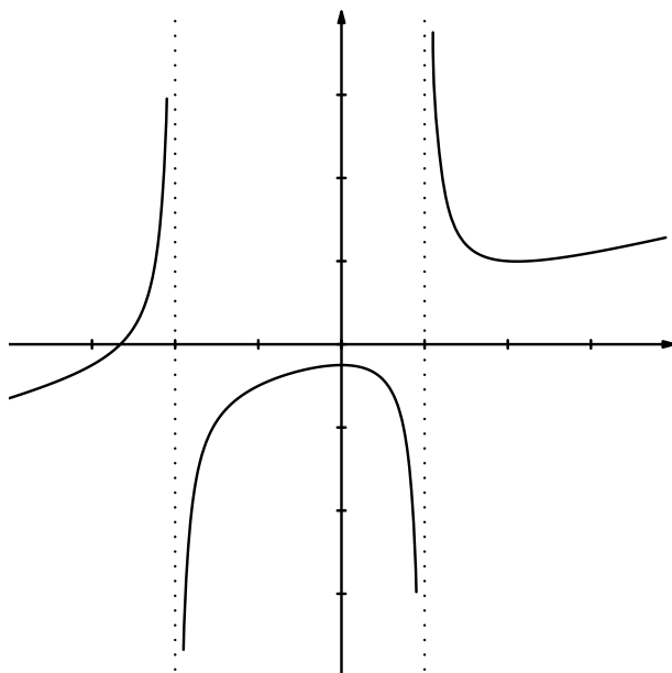
Figure 3.2: Przykład funkcji wymiernej.
