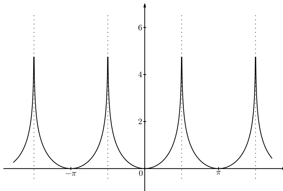
Figure 9.1: Wykres funkcji f(x) = -\log |\cos x| .
