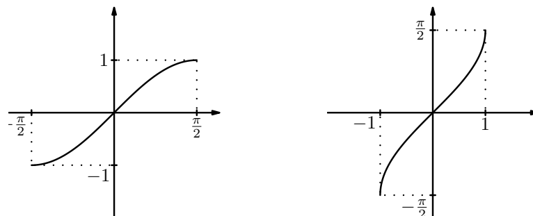
Figure 7.2: Funkcja \sin(x) i \arcsin(x) .
