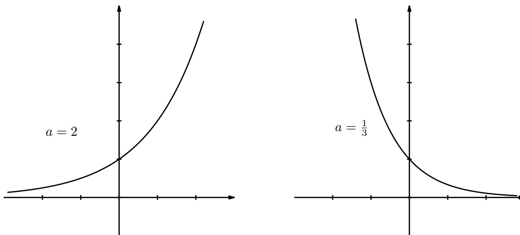
Figure 3.4: Funkcja wykładnicza f(x) = a^x .
