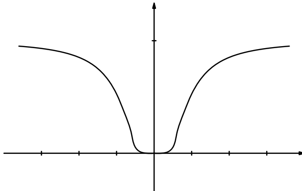
Figure 15.1: Funkcja z przykładu (c).
