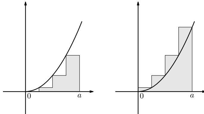
Figure 10.2: Mniejszy wielokąt i większy wielokąt.
