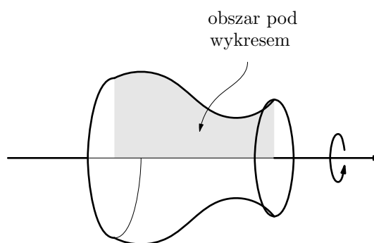
Rysunek 11.3: Bryła obrotowa.
