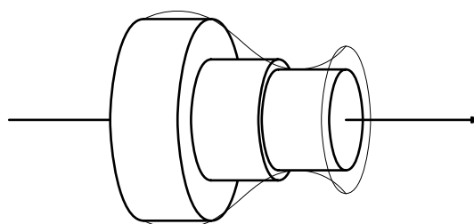
Rysunek 11.4: Przybliżanie objętości walcami.
