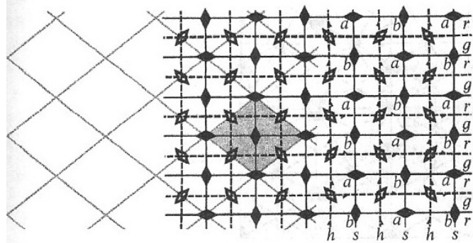
cmm
