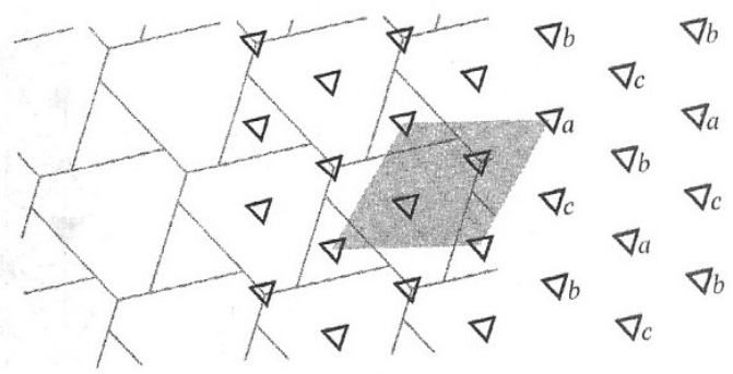
p3
