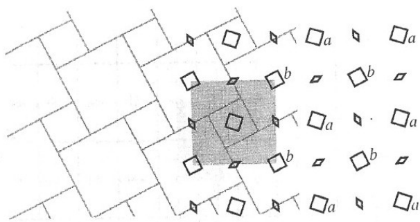
p4
