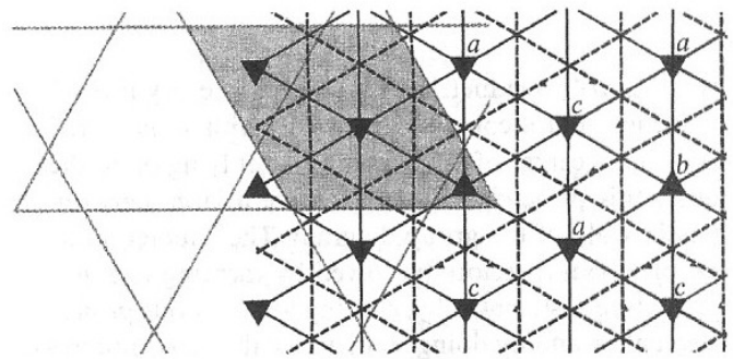
p3ml
