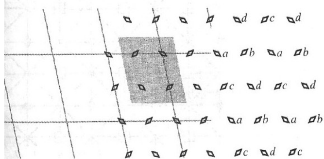
p2
