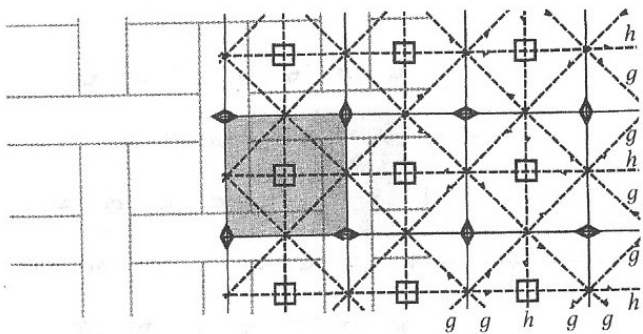
p4g
