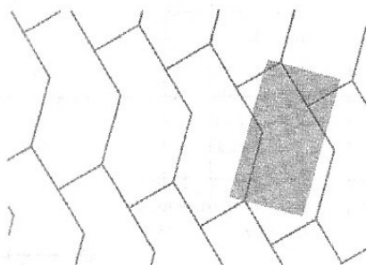
p1
